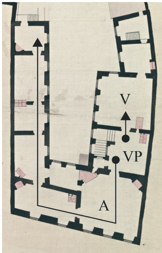
7. Antano Tyzenhauzo mūrnamio pirmo aukšto planas: VP – vestibulis-prieškambaris; V – valgomasis, A – vėliavininko A. Tyzenhauzo apartamentas, VUB RS F78-978, l. 2, detalė
