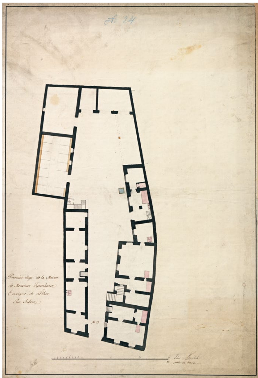
3. Tyzenhauzų namo Vilniuje, Subačiaus gatvėje projektas, pirmas aukštas ir kiemas su tarnybinėmis patalpomis, virtuve, arklidėmis ir kitomis ūkinėmis patalpomis, VUB RS, f. 78–978, l. 2
